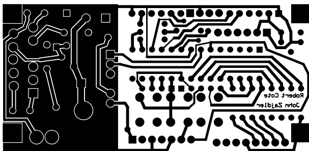
BOTTOM LAYER
