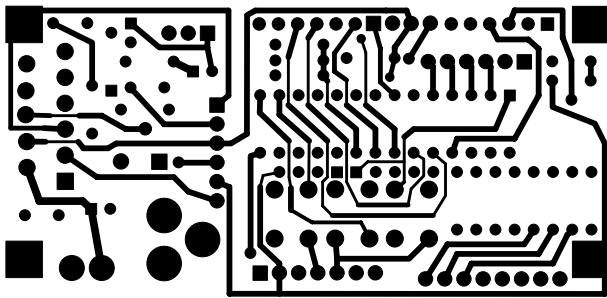
TOP LAYER
