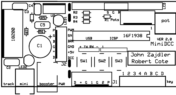
TOP OVERLAY
